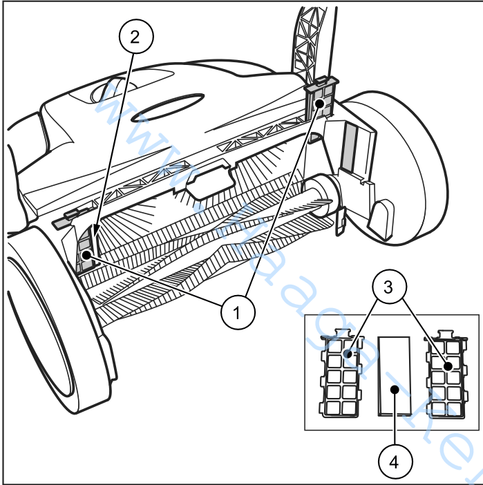
Abb. 12: Staubfilterentnahme
