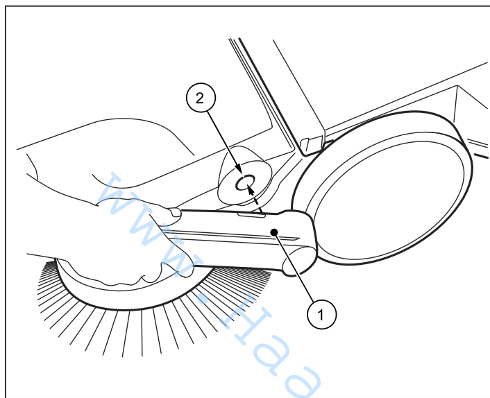
Abb. 7: Griffbeschlagmontage (haaga 375)
