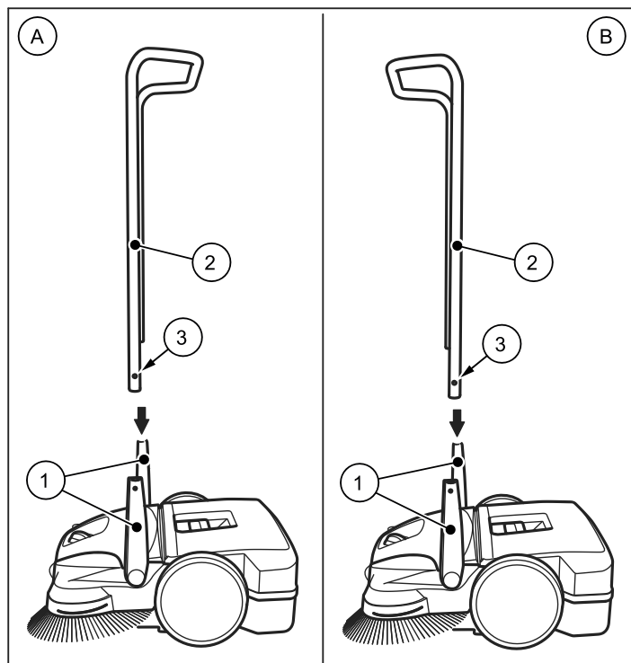
Abb. 8: Schiebebügelmontage
