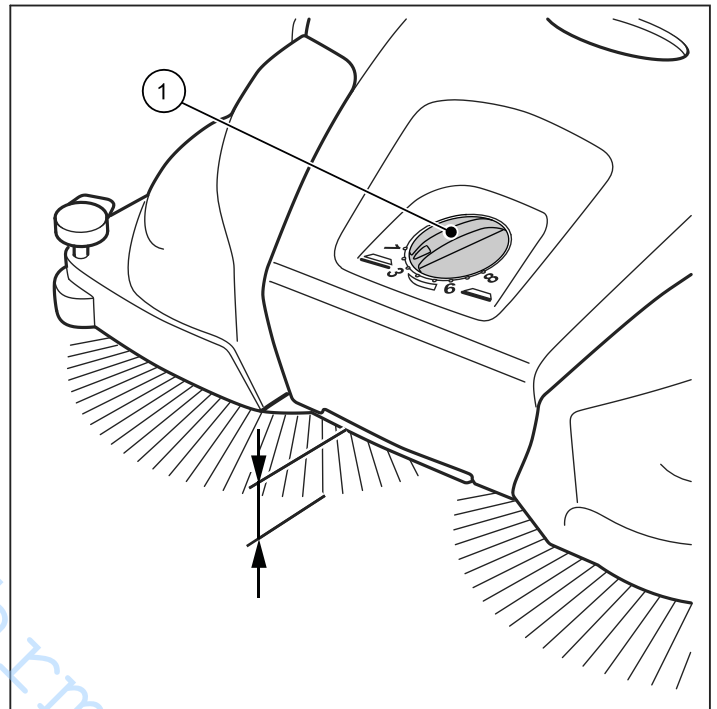
Abb. 9: Höhenverstellung Tellerbesen
